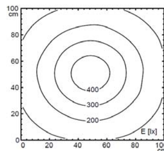
Lichtverteilung
